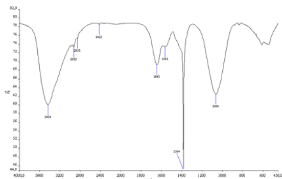
Fig. 1. FT-IR spectrum of Met x -EPS
