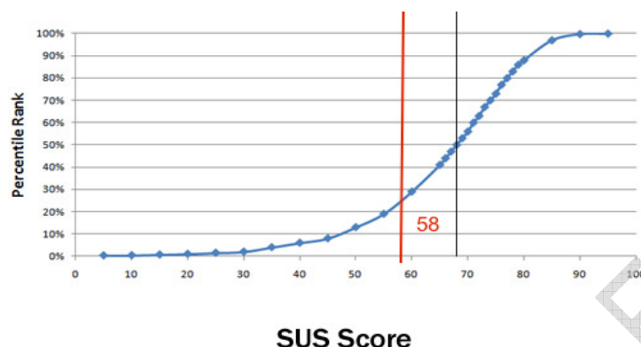
Fig. 3. SUS diagram for Website-2.
