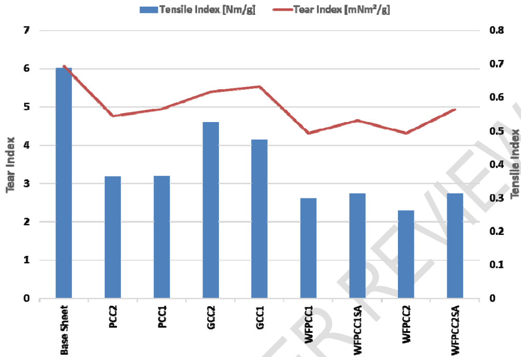
277 Fig. 7. Tensile / Tear 15% filler + WF
