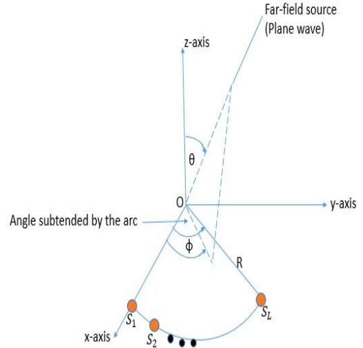
Fig. 2. Uniform Arc Array (UAA).
